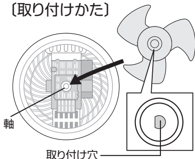
①軸と取り付け穴を 合わせて羽根を取り付ける
