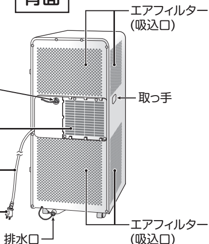
背面
