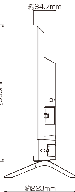
【本体右側面】
