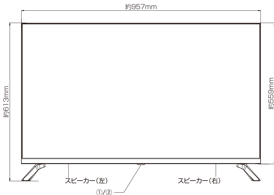
【本体前面】
