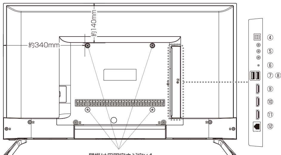
【本体背面】
