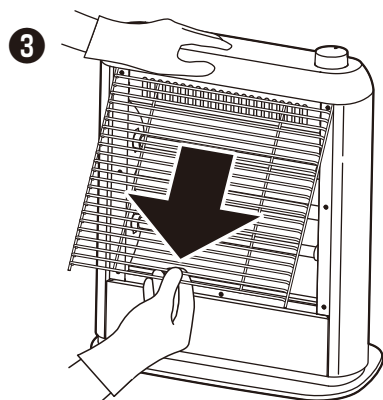
ガードを斜め下に引き抜く
