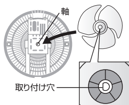
⑤羽根の取り付け穴(上図)の向きに注意しながら、軸と取り付け穴を合わせて羽根を取り付け、スピナーを左に回し羽根を固定する
