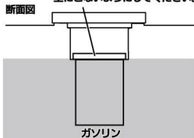
給油限界位置 ※プラスチックの部分より燃料が上にこないようにしてください。
