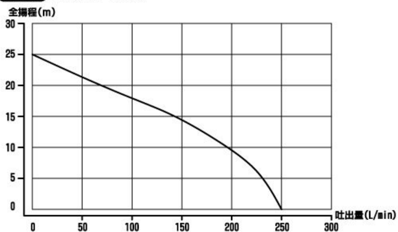
性能曲線 ※φ38mmホース使用時
