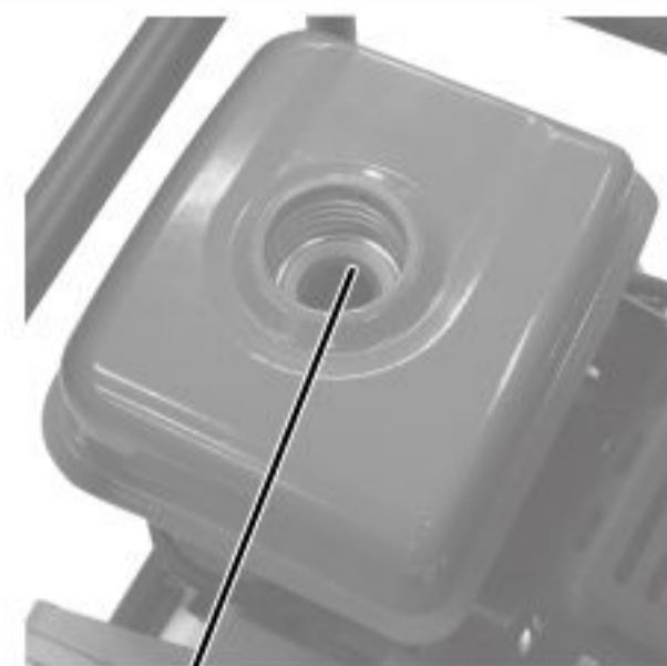
給油限界位置 ※プラスチックの部分より燃料が上にこないようにしてください。
