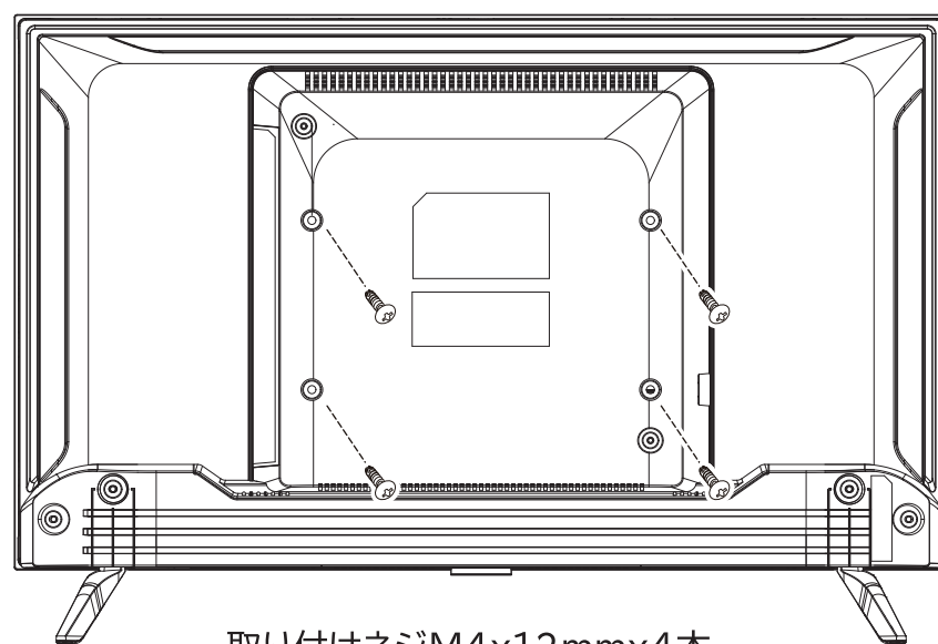
取り付けネジM4x12mmx4本
