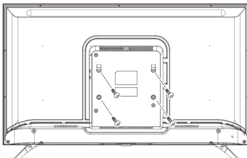
取り付けネジM6×10mm×4本
