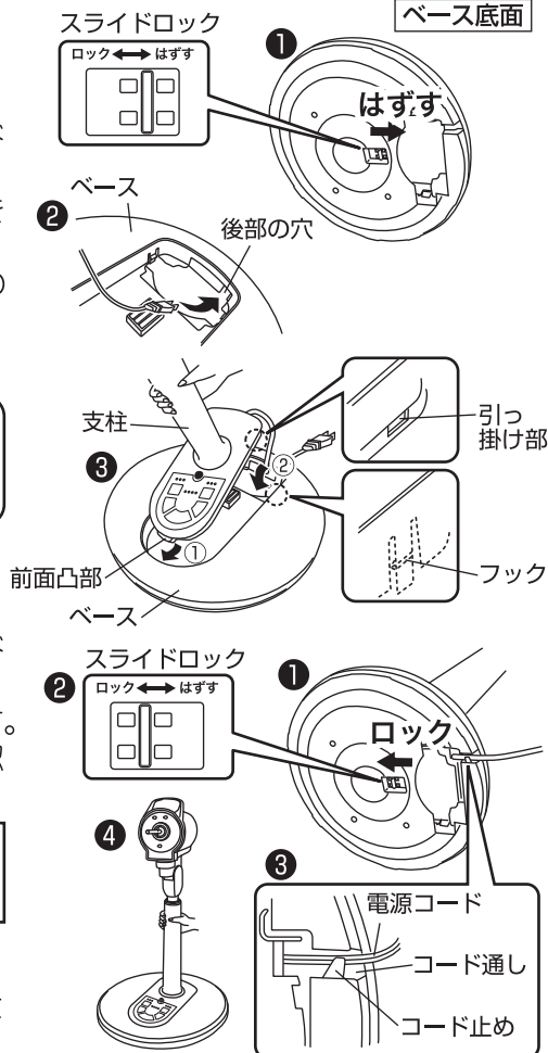
ベース底面
