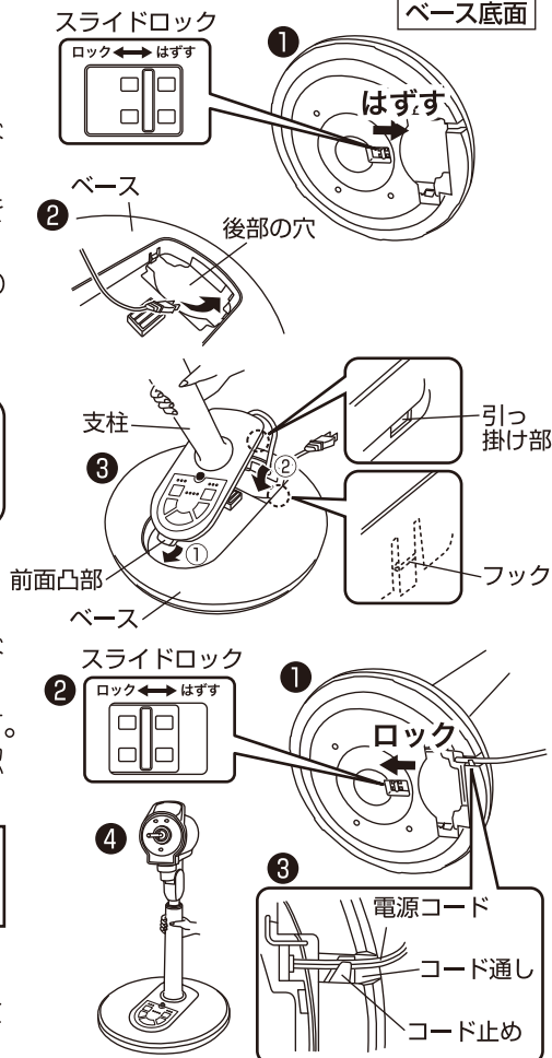
ベース底面
